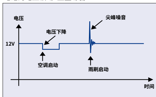
电池的电压波动·重叠噪音
