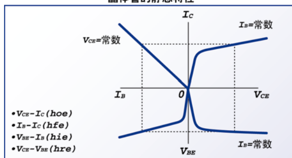
晶体管的静态特性
